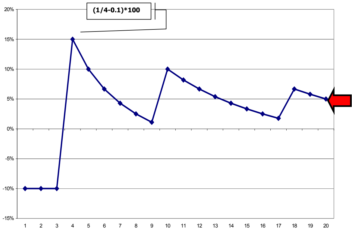
Figura 5. Differenza della probabilità osservata rispetto a quella attesa (10%)
