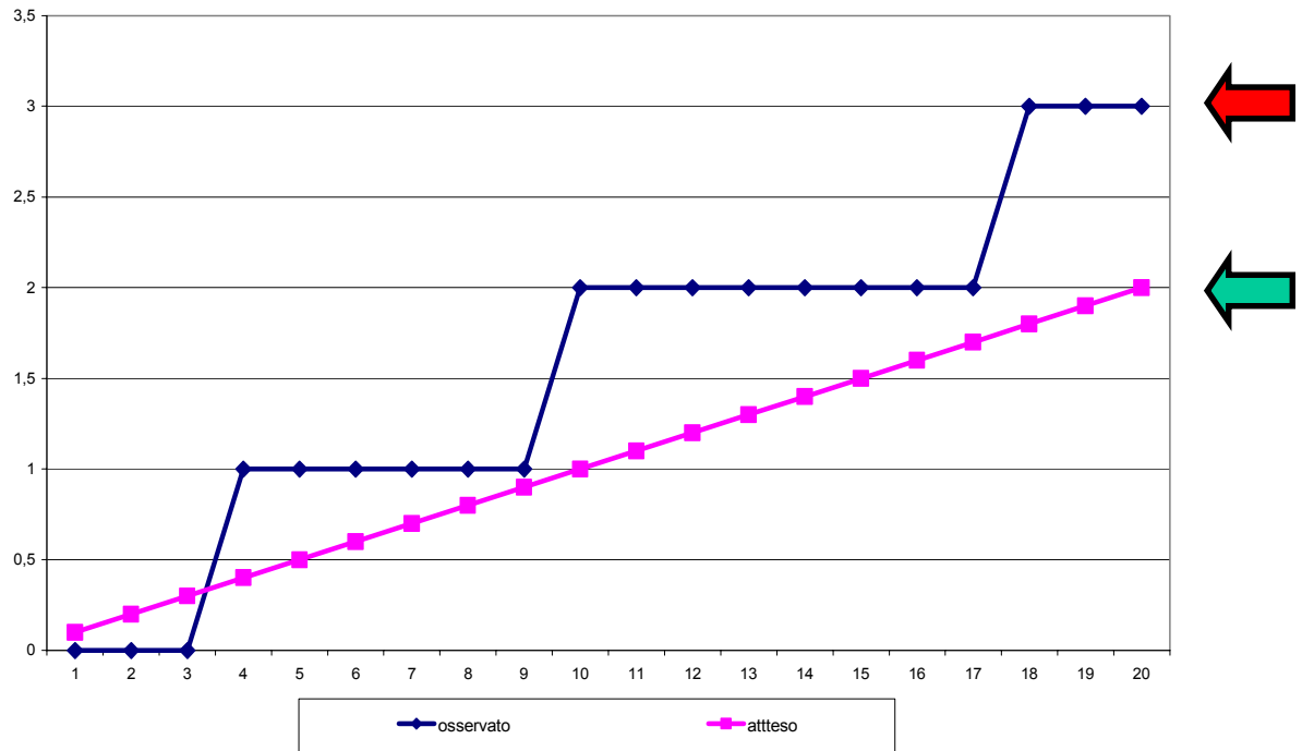
Figura 2. Grafico cumulata atteso e osservato
