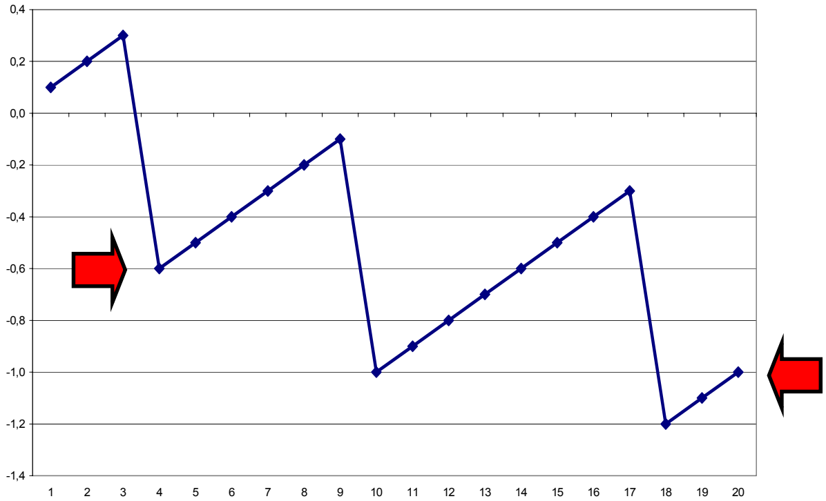
Figura 4. Spezzata differenza cumulata atteso e osservato
